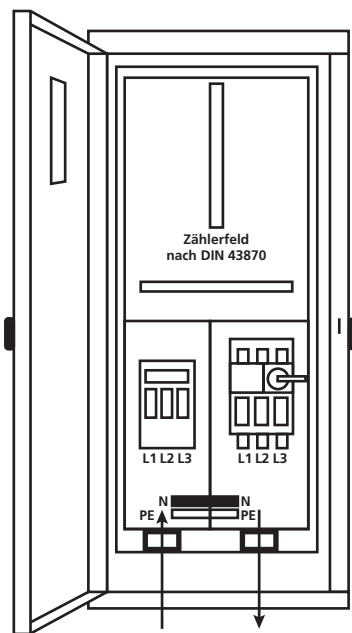
Anschlusschrank (Standardschrank)
