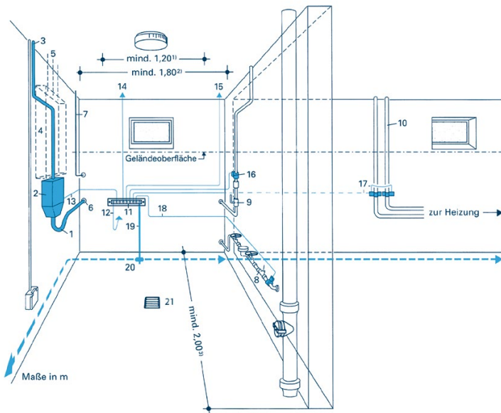
Abb. 1: Beispiel eines Hausanschlussraumes mit Hauptpotentialausgleich
